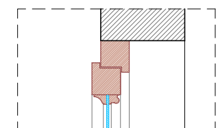
Particolare 2 Scala 1:10
