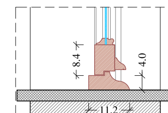
Particolare 3 Scala 1:10
