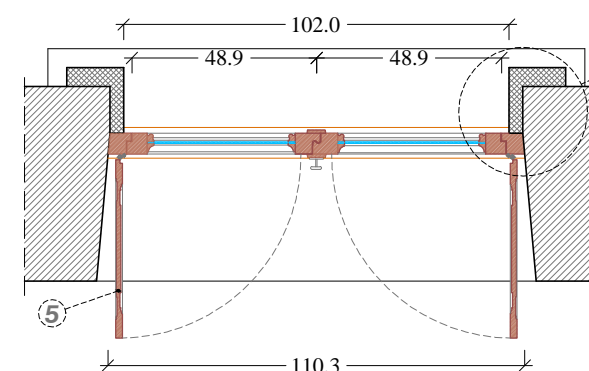
Sezione Orizzontale Scala 1:20
