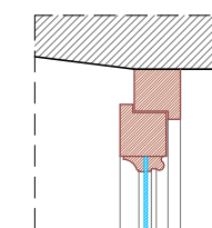
Particolare 2 Scala 1:10
