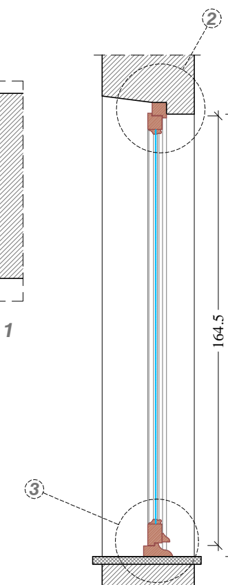
Sezione Verticale Scala 1:20
