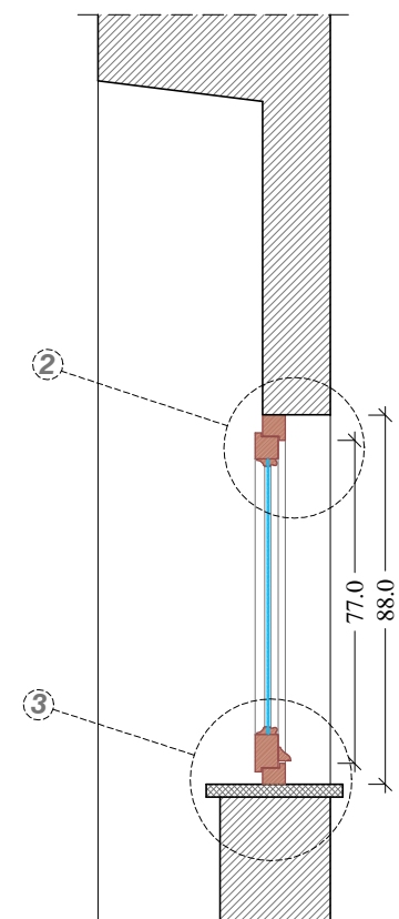
Particolare 2 Scala 1:10
