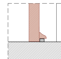
Particolare 4 Scala 1:10
