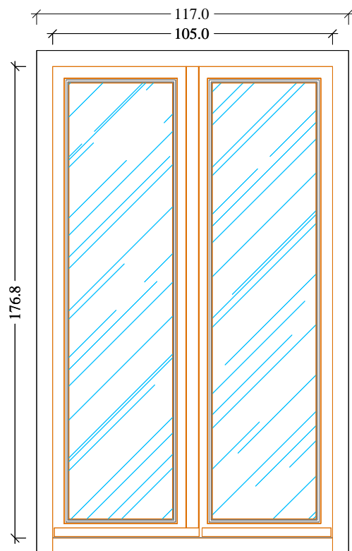
Prospetto Esterno Scala 1:20
