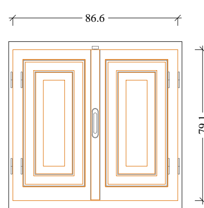
Scuri (vista interna) Scala 1:20
