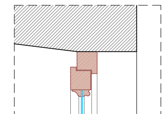
Particolare 2 Scala 1:10
