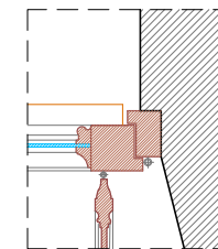
Particolare 1 Scala 1:10
