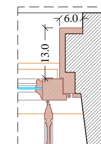
Particolare 1 Scala 1:10
