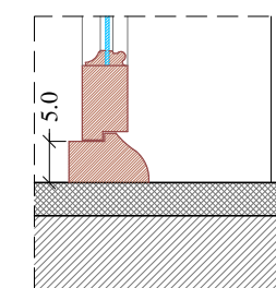
Particolare 4 Scala 1:10
