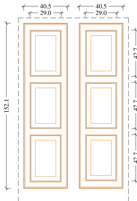
Scuri (vista esterna) Scala 1:20
