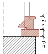
Particolare 2 Scala 1:10
