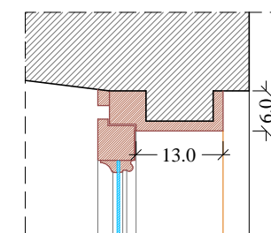
Particolare 2 Scala 1:10
