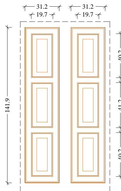
Scuri (vista esterna) Scala 1:20
