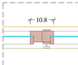
Particolare 5 Scala 1:10
