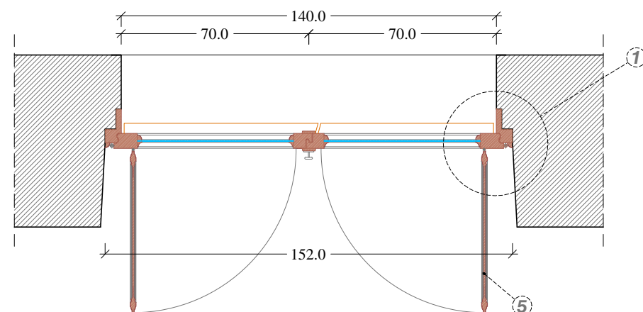
Sezione Orizzontale Scala 1:20
