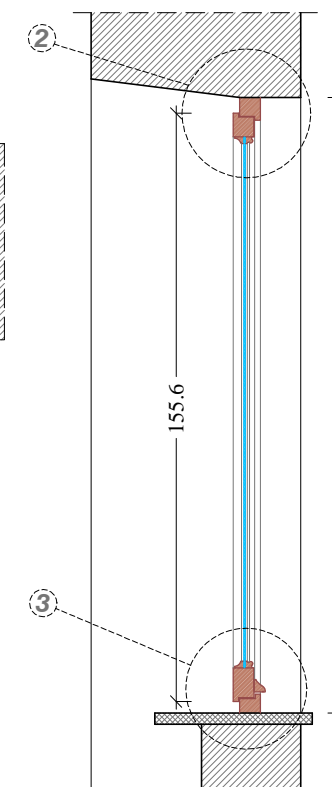
Sezione Verticale Scala 1:20
