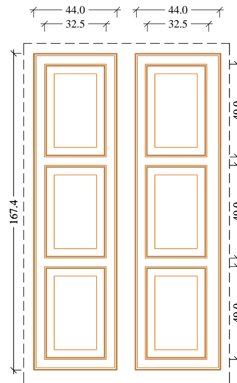
Scuri (vista esterna) Scala 1:20
