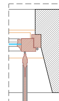
Particolare 1 Scala 1:10
