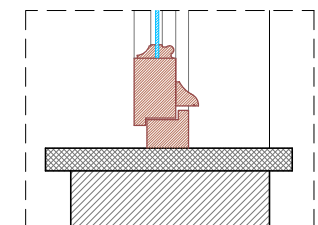
Particolare 3 Scala 1:10
