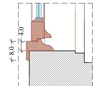
Particolare 3 Scala 1:10
