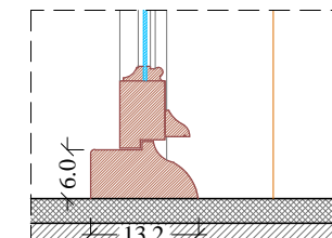
Particolare 3 Scala 1:10
