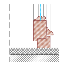
Particolare 3 Scala 1:10
