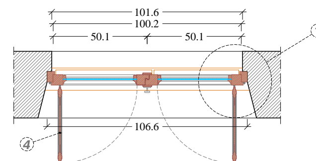
Sezione Orizzontale Scala 1:20
