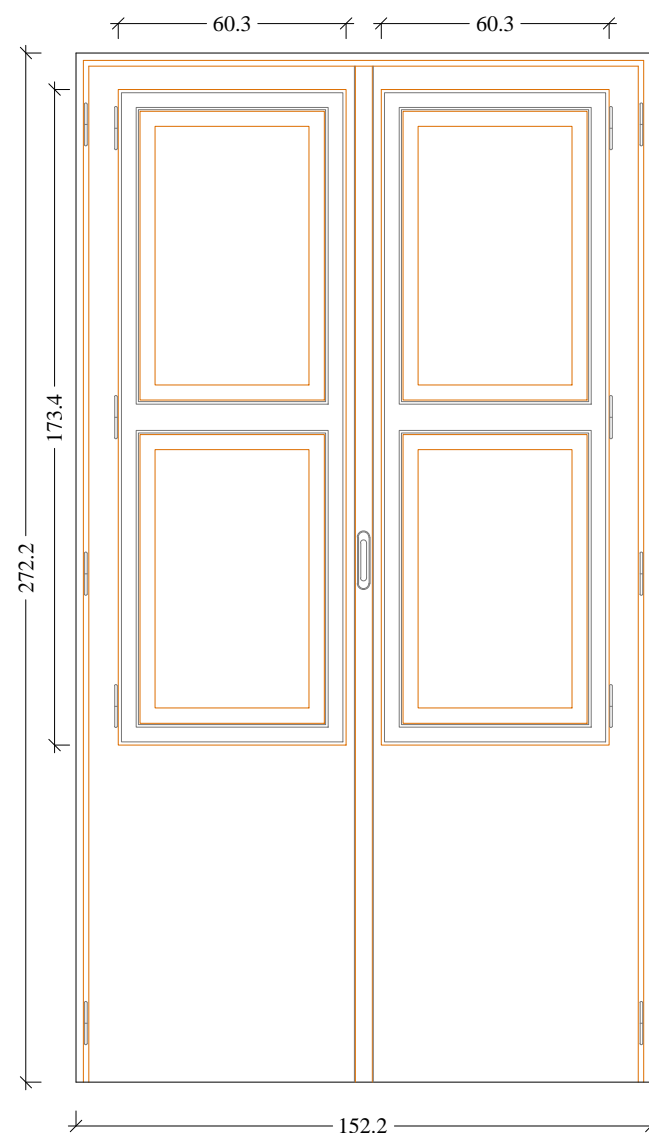
Scuri (vista interna/esterna) Scala 1:20
