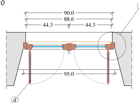
Sezione Orizzontale Scala 1:20
