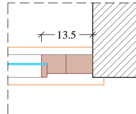
Particolare 3 Scala 1:10
