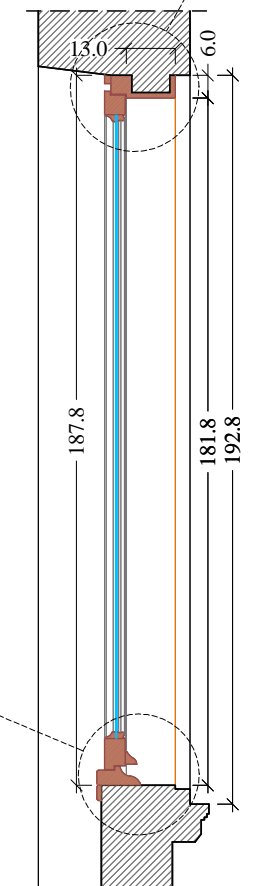
Particolare 2 Scala 1:10
