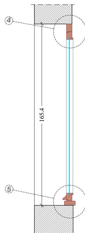
Particolare 1 Scala 1:10
