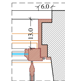
Particolare 1 Scala 1:10
