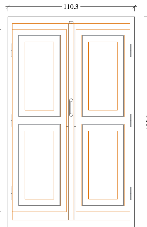
Scuri (vista interna) Scala 1:20
