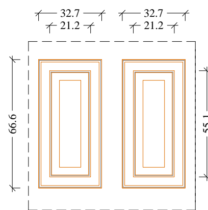
Sezione Orizzontale Scala 1:20
