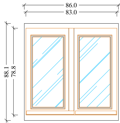
Prospetto Esterno Scala 1:20
