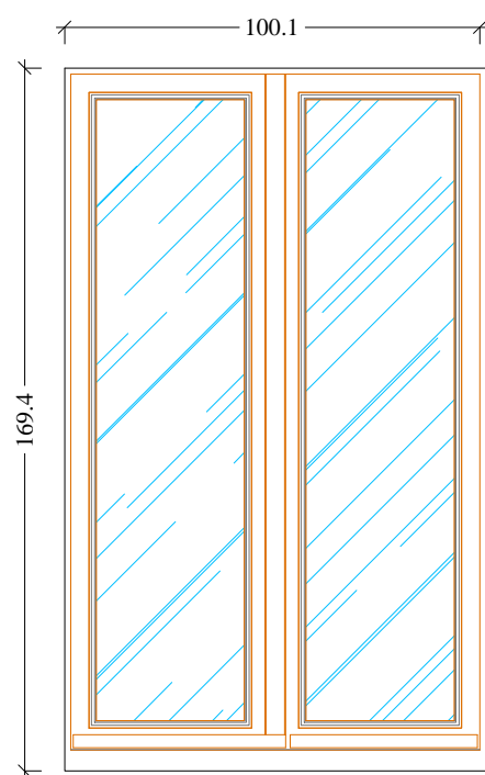
Prospetto Esterno Scala 1:20
