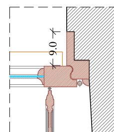
Particolare 1 Scala 1:10
