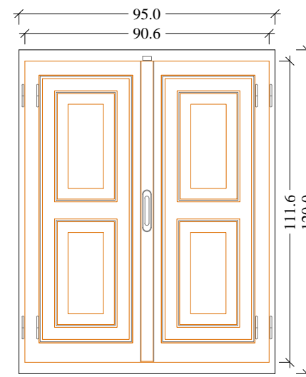
Scuri (vista interna) Scala 1:20
