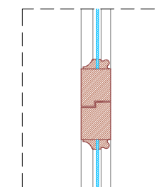
Particolare 3 Scala 1:10
