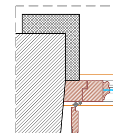
Particolare 1 Scala 1:10
