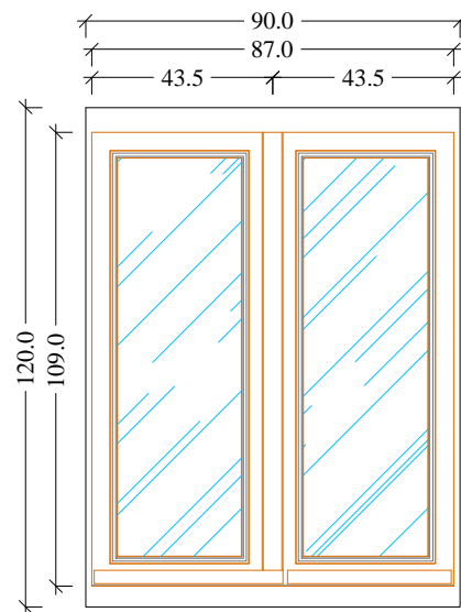
Prospetto Esterno Scala 1:20
