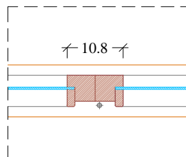
Particolare 4 Scala 1:10
