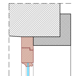
Particolare 2 Scala 1:10
