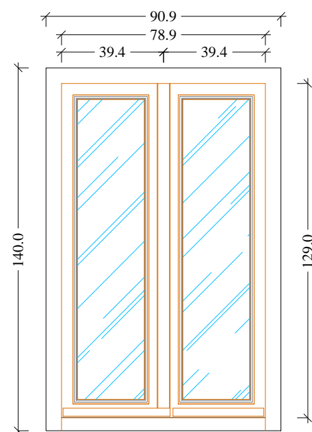
Prospetto Esterno Scala 1:20
