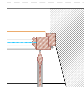
Particolare 1 Scala 1:10
