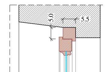
Particolare 2 Scala 1:10
