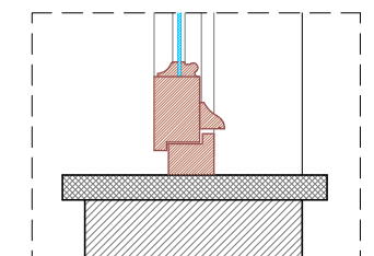
Particolare 3 Scala 1:10
