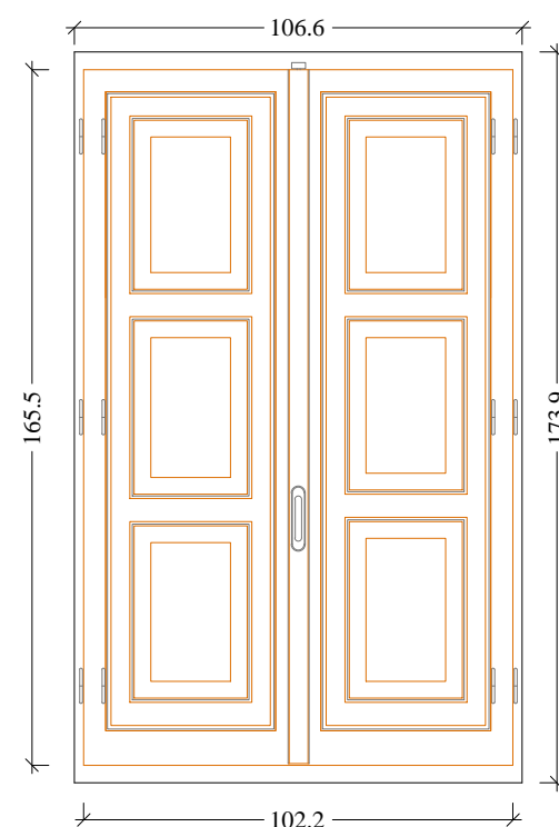
Scuri (vista interna) Scala 1:20
