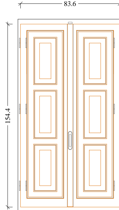
Scuri (vista interna) Scala 1:20
