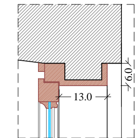
Particolare 3 Scala 1:10
