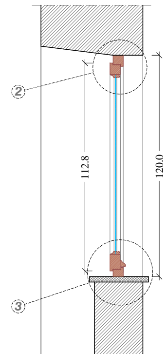
Sezione Verticale Scala 1:20
