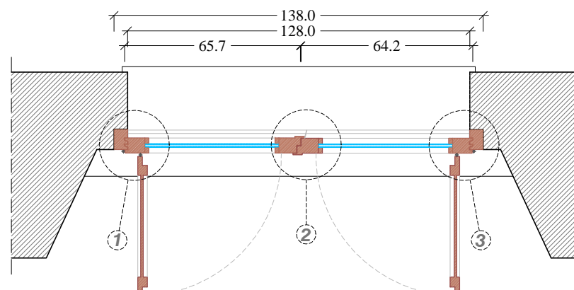
Sezione Orizzontale Scala 1:20
