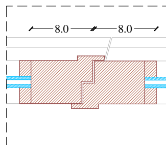
Particolare 2 Scala 1:5
