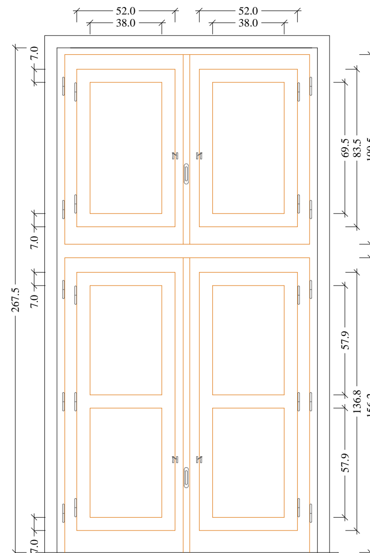
Scuri (vista interna) Scala 1:20
