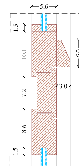
Particolare 5 Scala 1:5
