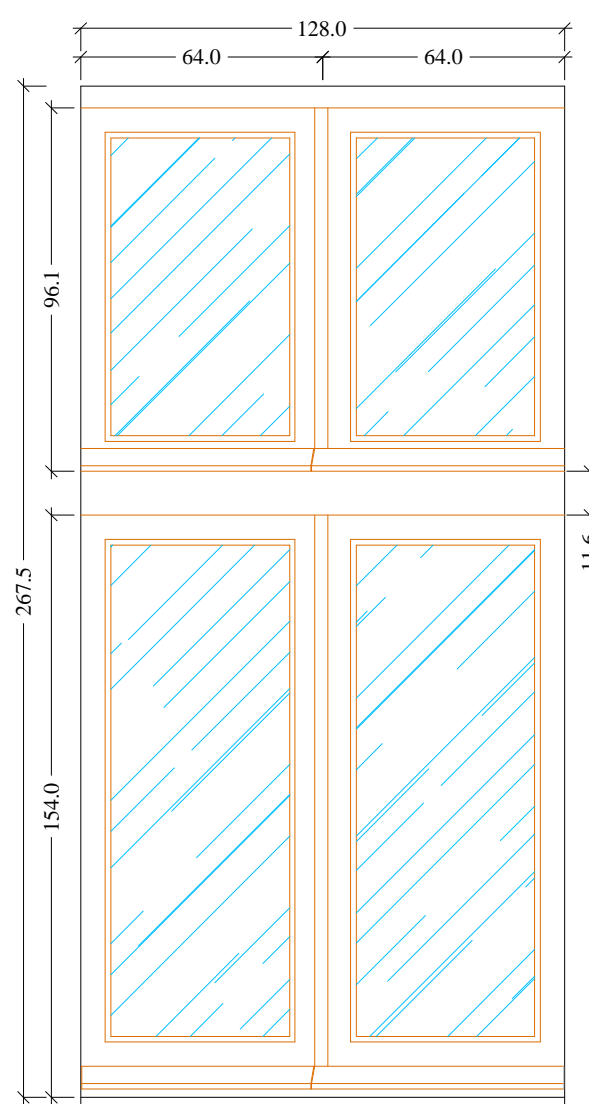
Prospetto Esterno Scala 1:20
