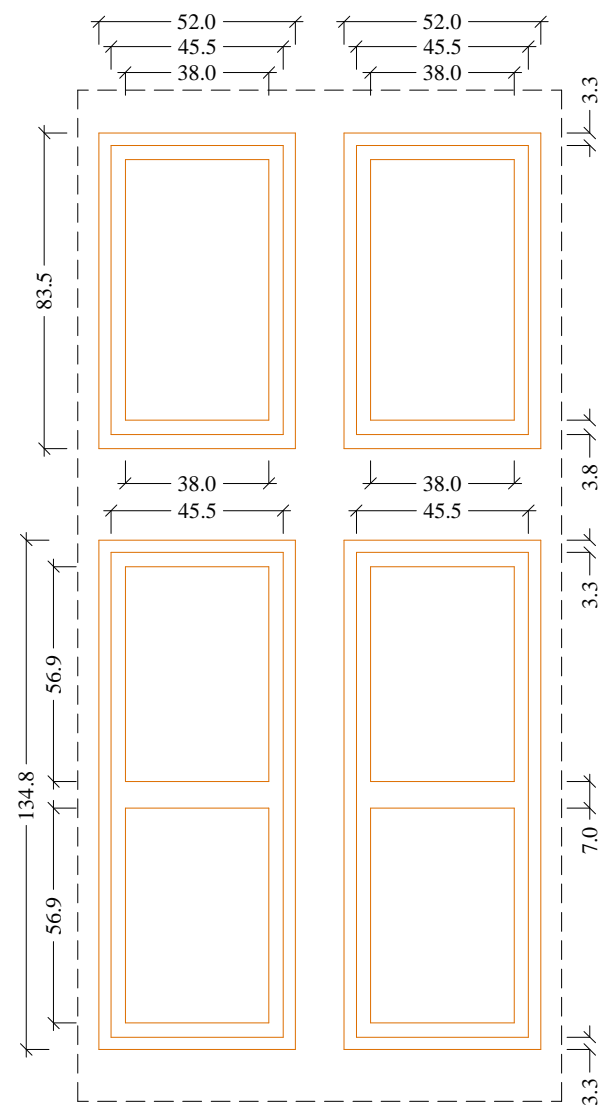
Scuri (vista esterna) Scala 1:20
