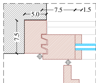
Particolare 1 Scala 1:5
