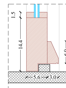
Particolare 4 Scala 1:5
