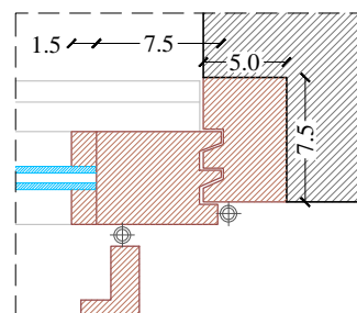
Particolare 3 Scala 1:5
