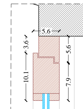
Particolare 6 Scala 1:5
